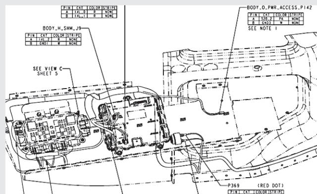
Intérieur du compartiment d'interrupteurs situé à gauche du conducteur (C2)
